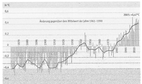
Entwicklung der globalen Mitteltemperatur 1861 - 2005 (Quelle: World Meteorological Organization)
